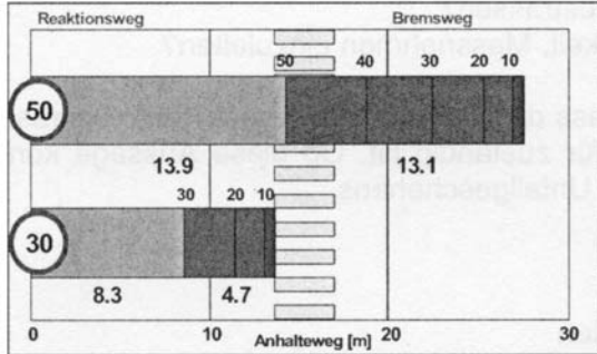
Abb. 1: Anhalteweg - Abbau der Geschwindigkeit auf trockener Strasse
